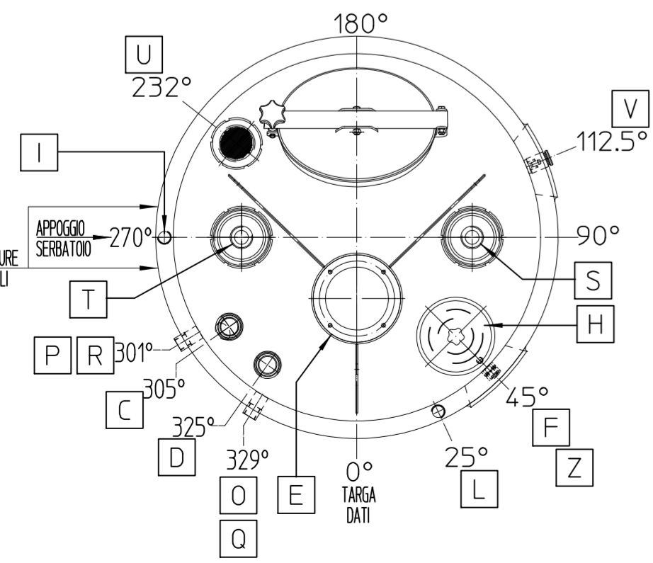
VISTA COPERCHIO DALL'ALTO
