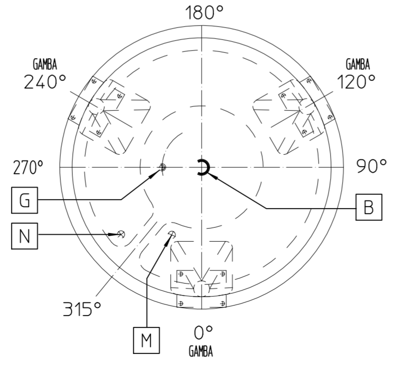
VISTA FONDO DALL'ALTO
